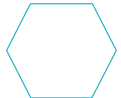
Hexágono
