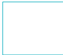
Cuadrado
